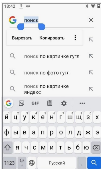
Рисунок 16. Копирование текста
