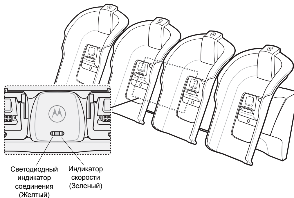
Рис. 8-7 Светодиодные индикаторы базовой станции Ethernet на 4 устройства
