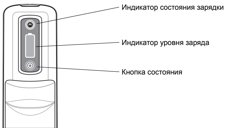
Рис. 2-1 Аккумулятор
