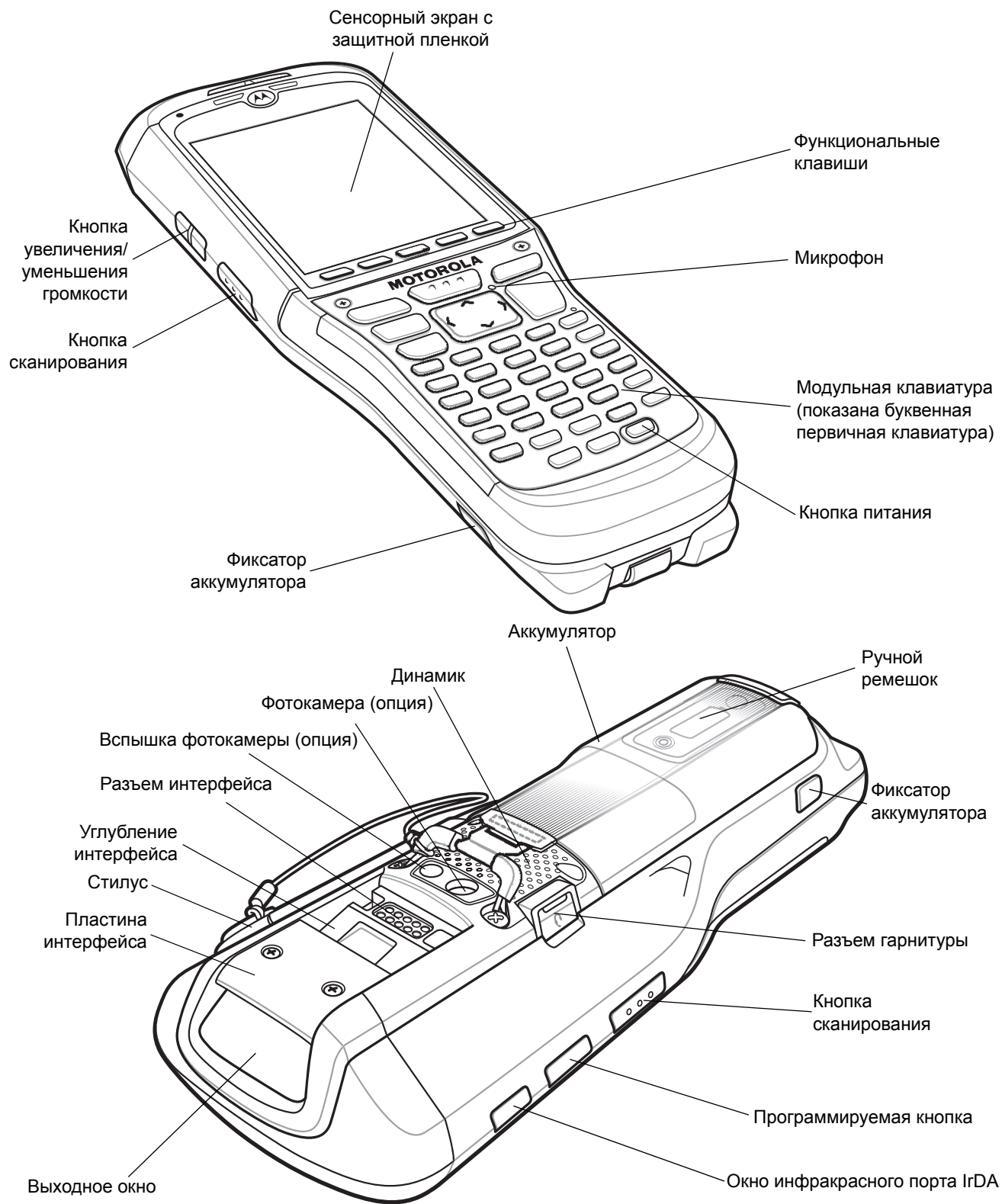
Рис. 1-1 MC9500-K
