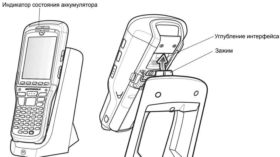
Рис. 8-2 Зарядка аккумулятора MC9500-K
