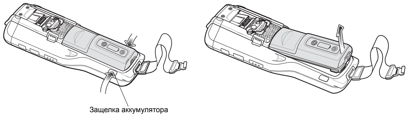
Рис. 1-9 Извлечение аккумулятора
