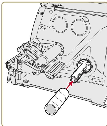
Закрепите подложку на картонной втулке рулона
