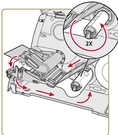
Закрепите подложку на картонной втулке рулона
