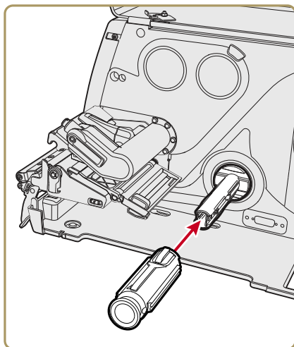
Закрепите подложку на разъемном стержне (PM43, PM43c)
