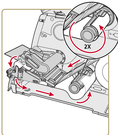
Закрепите подложку на разъемном стержне (PM43, PM43c)
