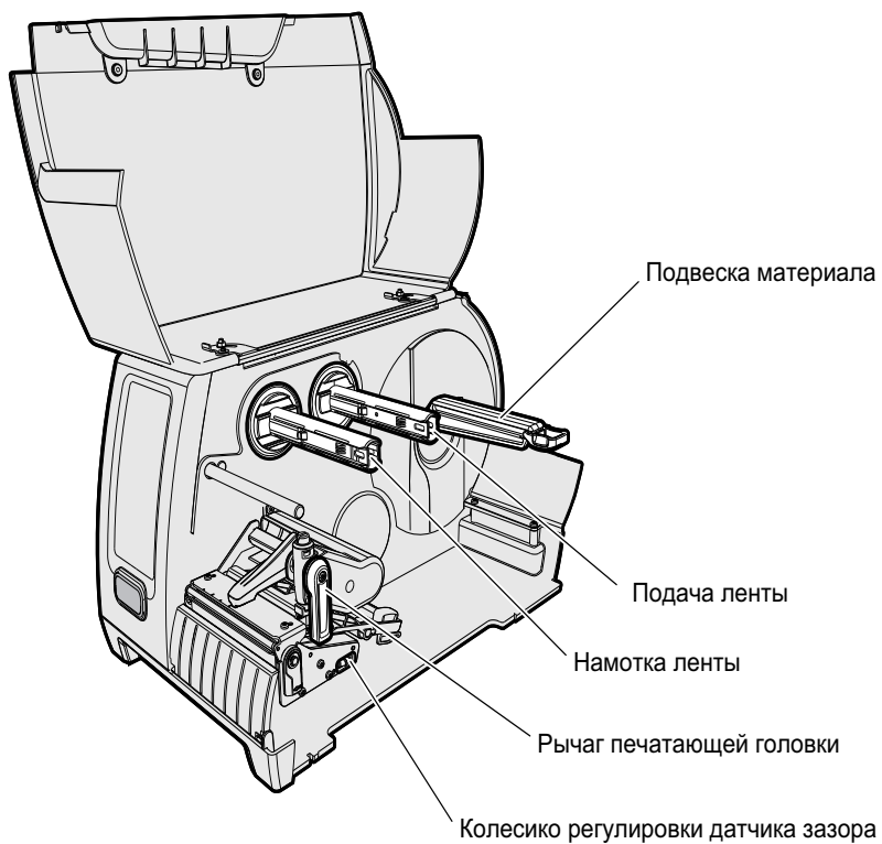
Вид изнутри принтера PM43
