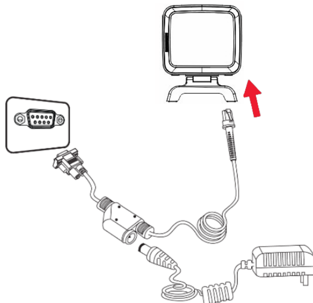
Рисунок 5. Подключение с помощью RS-232 кабеля
