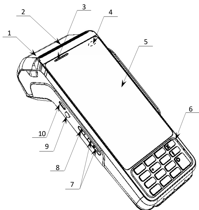
Рисунок 1. Вид сверху/спереди/слева
