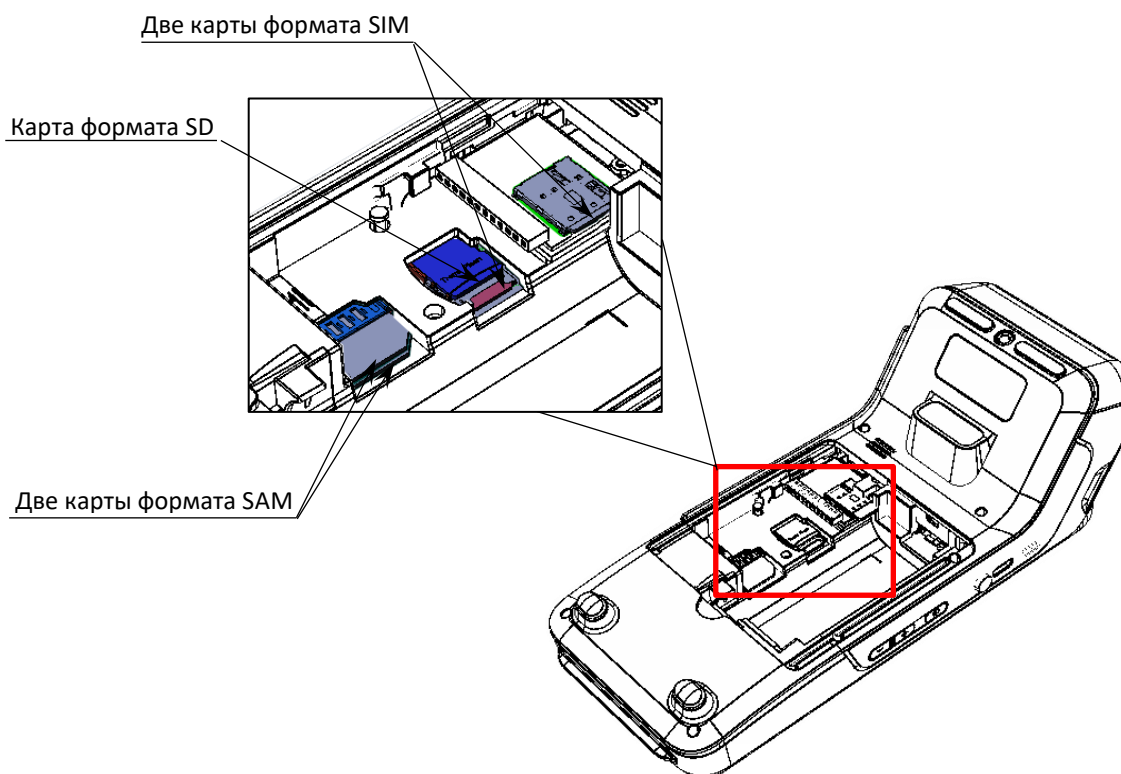
Рисунок 14. Расположение карт в корпусе ККТ
