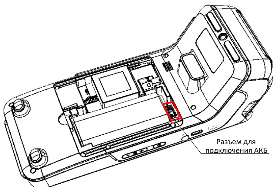
Рисунок 5. Расположение разъема для подключения АКБ
