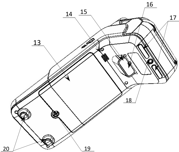
Рисунок 3. Вид снизу/сзади/справа
