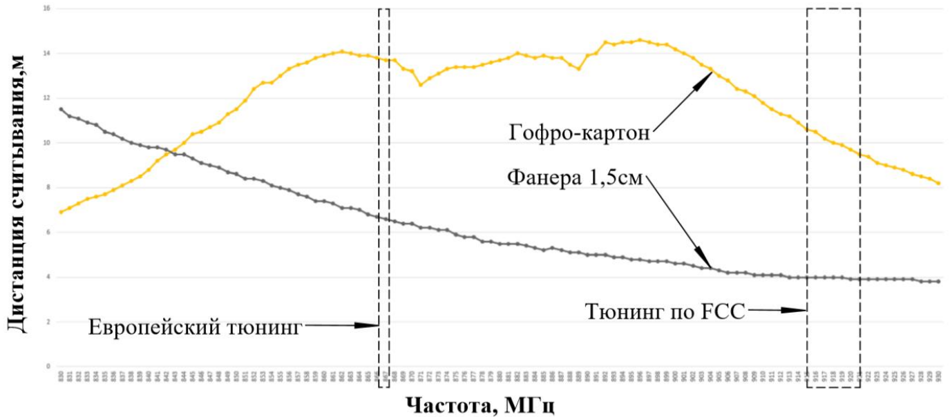
Рис.3 Дистанция считывания метки на фанере и картоне.
