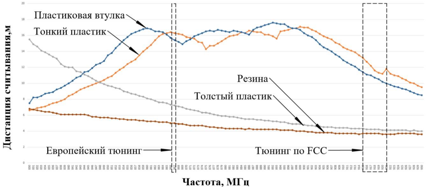
Рис.1 Дистанция считывания метки на резине и пластике.
