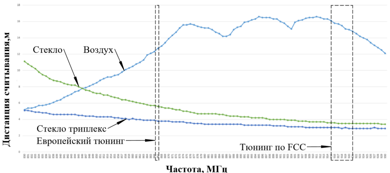
Рис.2 Дистанция считывания метки в воздухе и на стекле.
