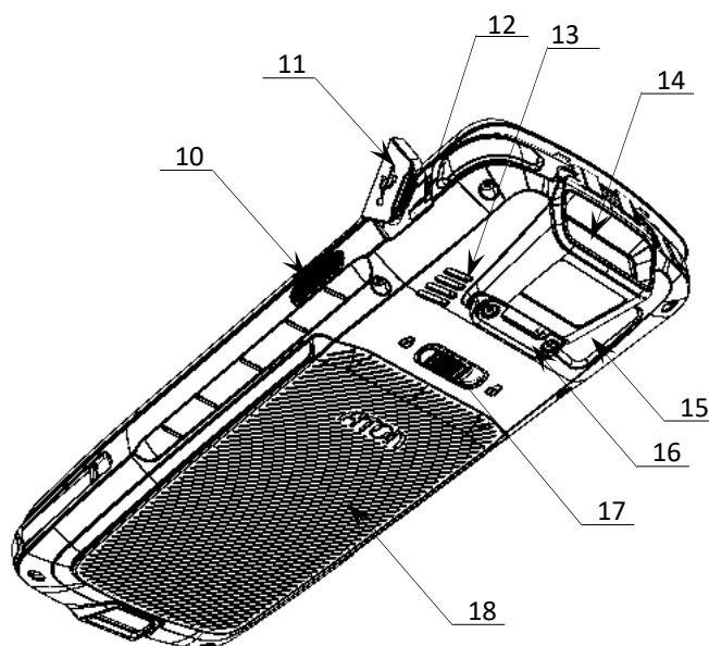
Рисунок 2. Вид сзади/справа
