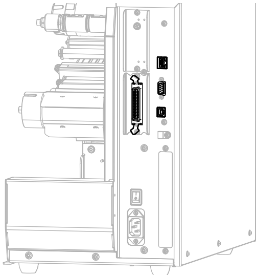
Рис. 18 Расположение интерфейсов обмена данными
