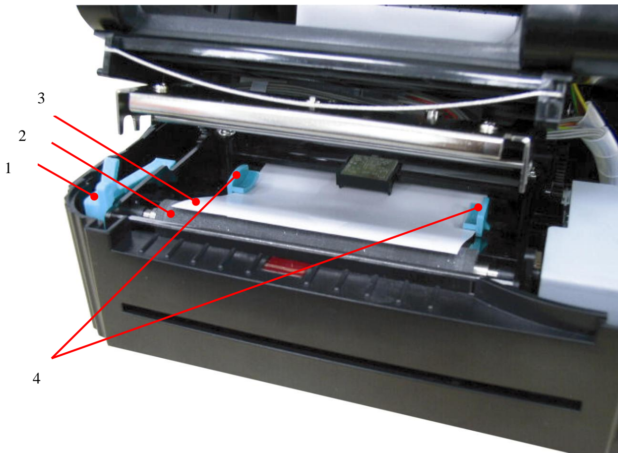
Рис. 6. Подача этикеток через регулирующую направляющую
