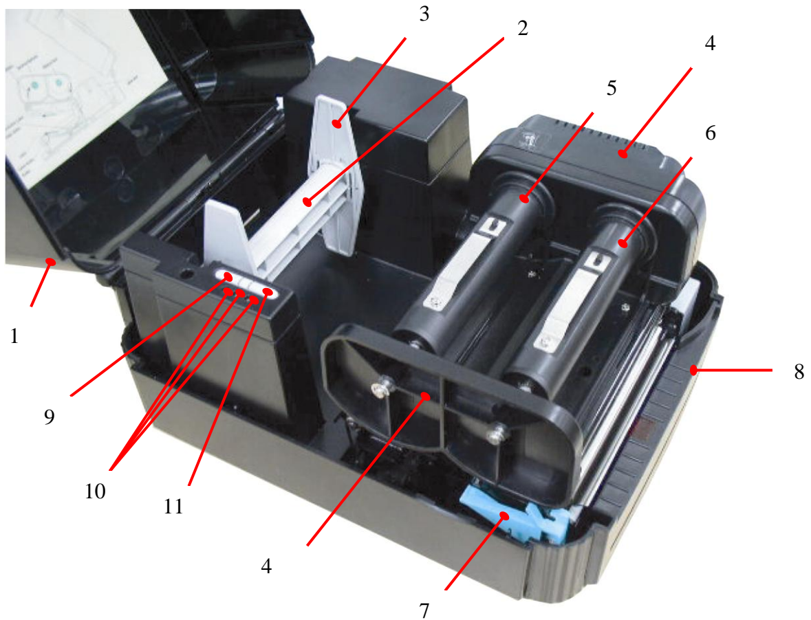
Рис. 2. Вид внутренних компонентов
